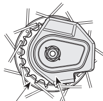
Piasta z wewnętrznymi przełozeniami Zespół silnika
